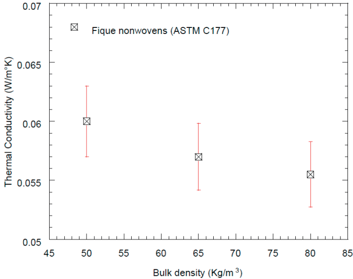
Conductividad térmica del fique Vs densidad del fique.
