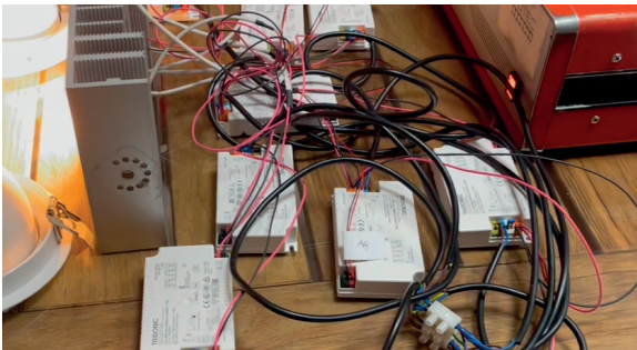
Luminaria desarrollada por el grupo de investigación.
