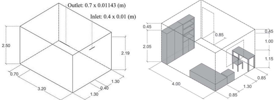
Disposiciones de la cámara de prueba (en metros) y disposiciones de entrada y salida del aire.
