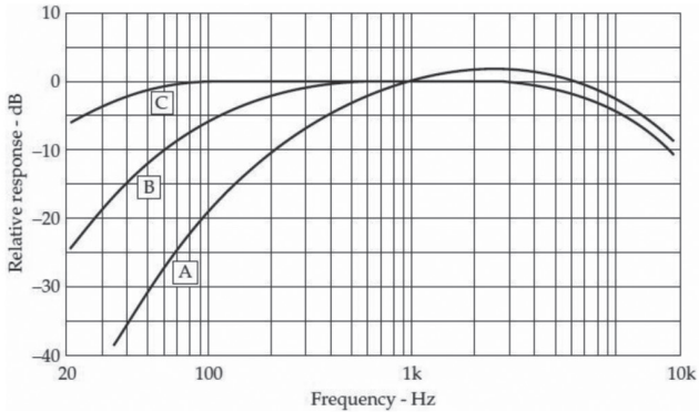
Filtro tipo A que casi anula las frecuencias audibles mas bajas.
