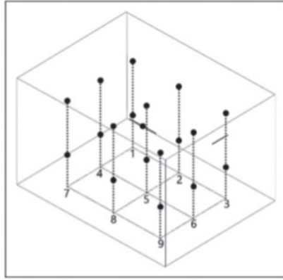
Distribución espacial de 9 puntos de medida a 0,75m y 2m.
