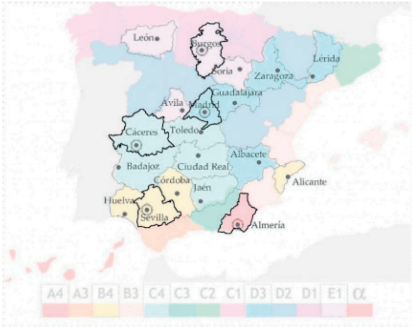
Zonas climáticas estudiadas de España.
