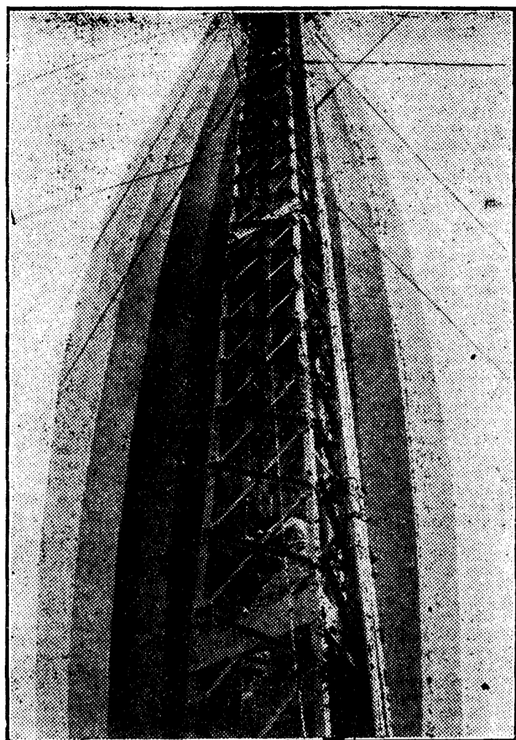
En el grabado de la izquierda se ve el interior del mástil de amarre con el dirigible, sujeto a él por la proa. Puede apreciarse el ascensor, que se utiliza para la carga y descarga, y que permite a la aeronave tomar pasajeros y mercancías sin necesidad de aterrizar. El otro grabado muestra al «R. 33», momentos antes de ser amarrado, al llegar al aeródromo de Pulham el día 2 de abril, procedente de Cardington, donde se habían hecho las reparaciones. En el gráfico hemos dibujado el camino probable del «R. 33» desde que fué arrastrado hasta que regresó a su base. En los rectángulos van indicadas las horas.
