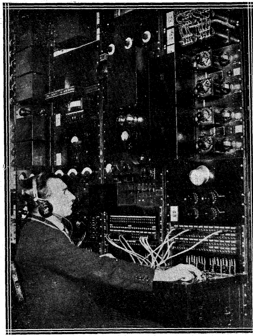
Instalación que se utilizara para la anunciada comunicación radiotelefónica entre Londres y Nueva York...
