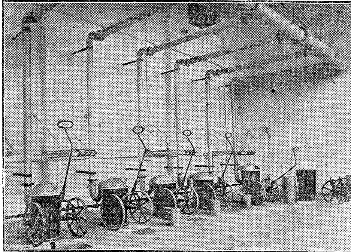
Los hornos de copales
