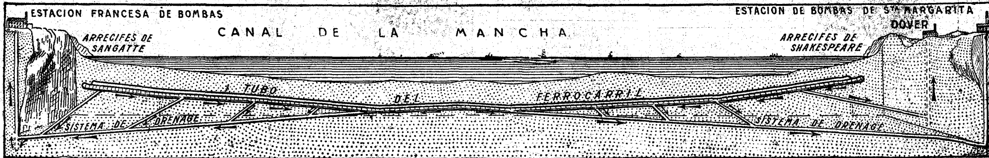
Proyecto de túnel bajo el Canal de la Mancha presentado doble túnel a 260 pies bajo el nivel del mar y 95 pies bajo el primer proyecto, cuya construcción llegó a iniciarse. Toda vía en Sangatte y Dover se conservan algunas instalaciones de 1875 y 1882.
