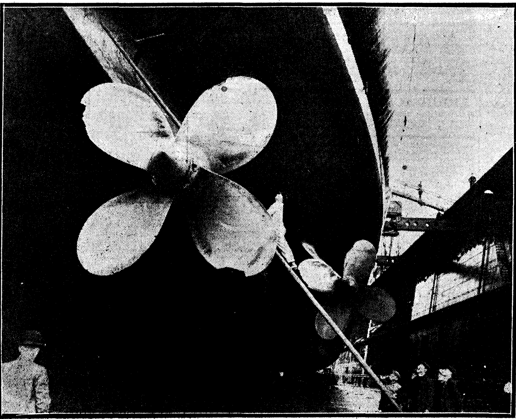
El "Bremen", el modernísimo buque alemán que batió el "record" de velocidad en el Atlántico, en el dique seco de Southampton. Un ingeniero examina las hélices. (Foto Vidal.)
