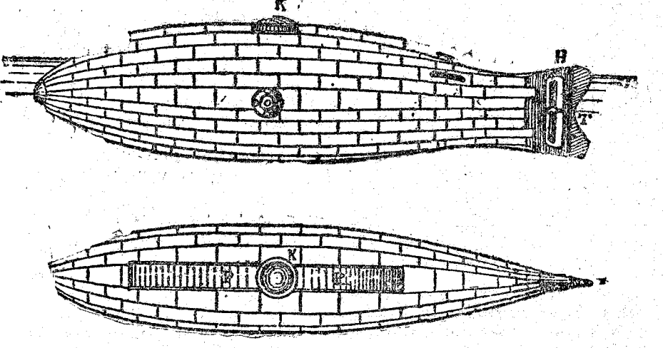
El «Ictíneo», ó barco pez, de Monturiol, según un dibujo del inventor.
