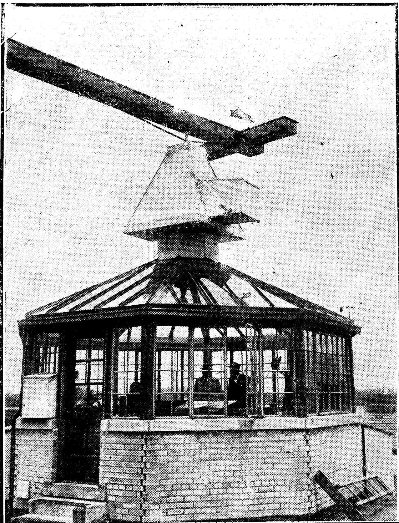
En el aerodromo de Cleveland se ha instalado esta torre, desde la cual se envían por "radio" a los aviadores todas las instrucciones para el aterrizaje. La posición de cualquier avión que se acerque al campo, es señalada automáticamente en el mapa que se ve en el interior (Fot. Vidal)
