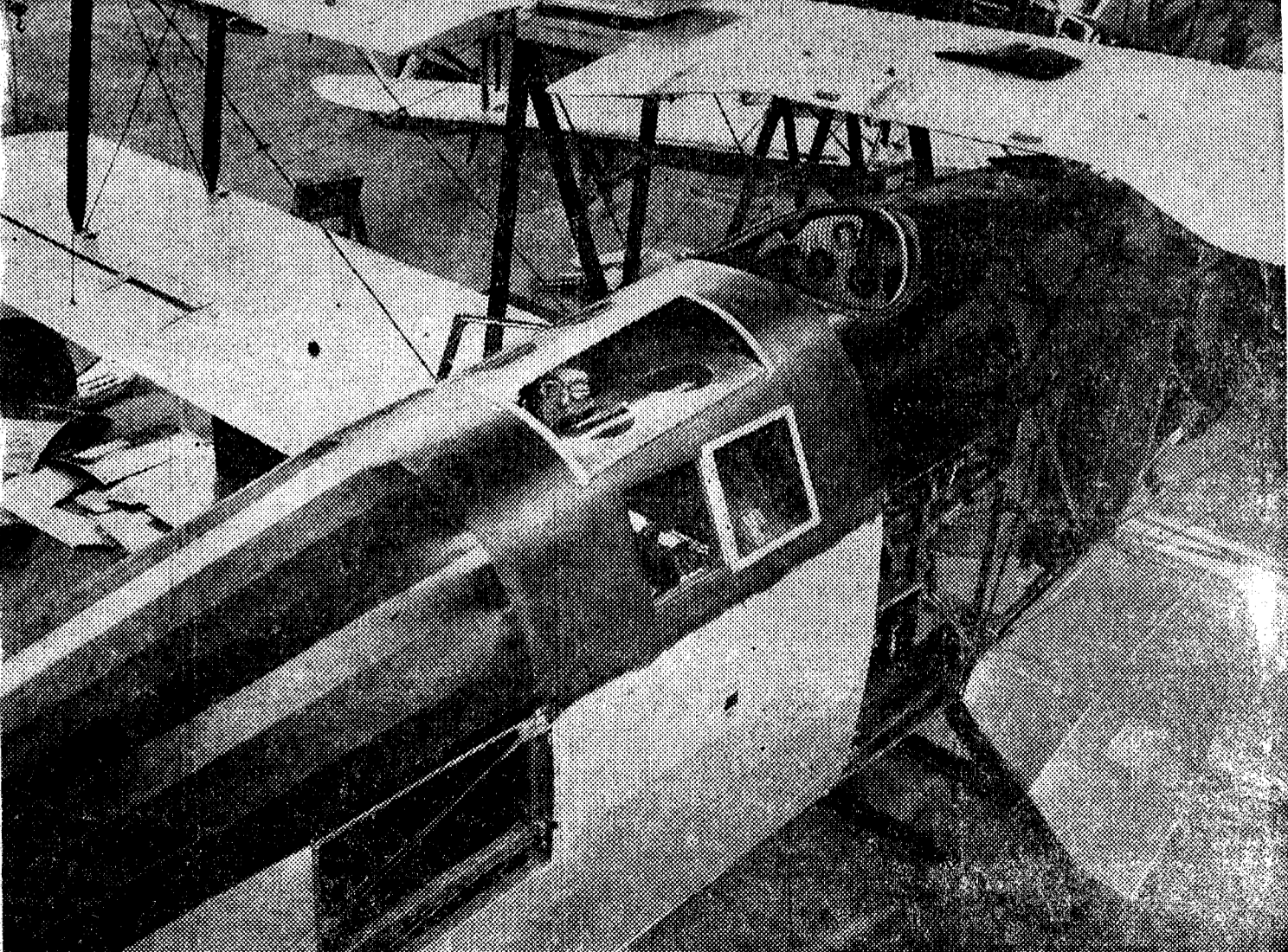
El puesto del observador va protegido contra el mal tiempo por un techo con ventanas. En las de los lados irán montadas las máquinas cinematográficas. El puesto del piloto va al descubierto
