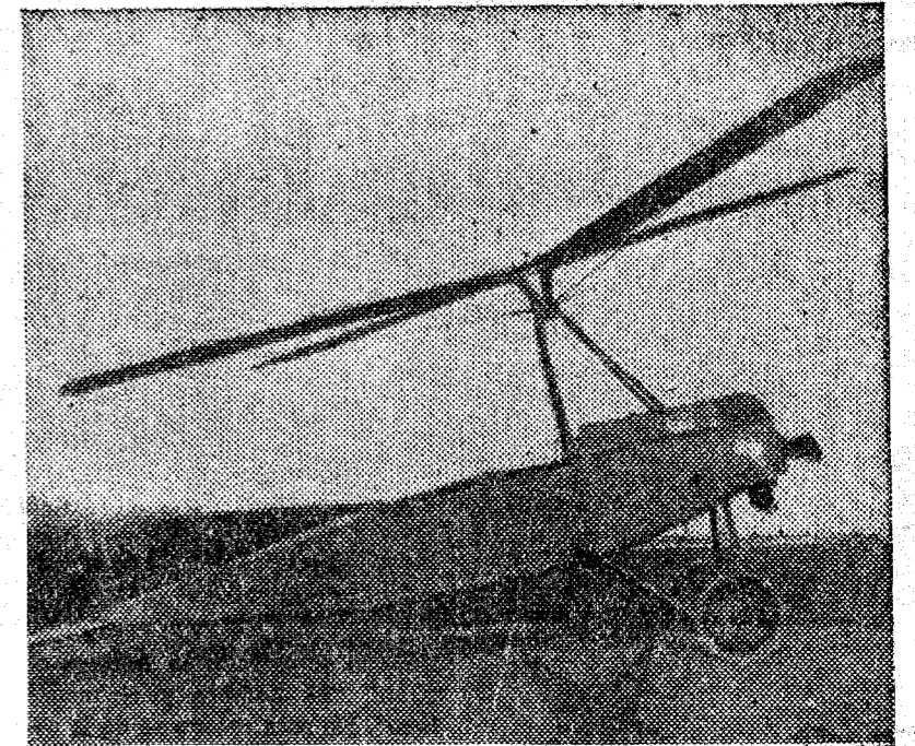
1923.—Primer autogiro que se elevó de tierra. Para conseguirlo, hubo que añadirle alas y otros elementos del avión. Múltiples problemas secundarios impiden volar sin alas
