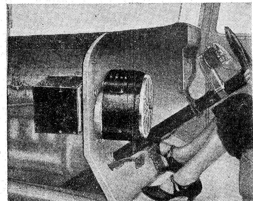
Equipo de Radio para automóvil de la Wells-Gardner, que presenta la Casa TELEAUDION, Eduardo Dato, número 11, especializada en estas instalaciones
