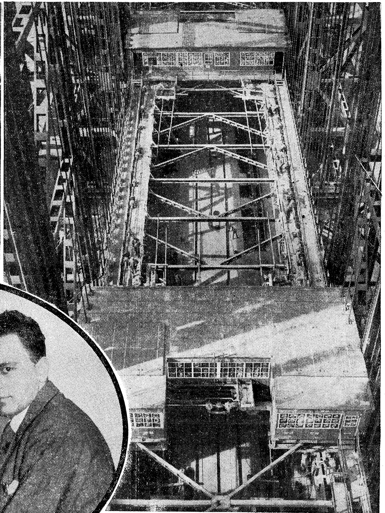
Vista parcial del elevador gigante de barcos que se está construyendo en Eilerswalde, al norte de Berlín
