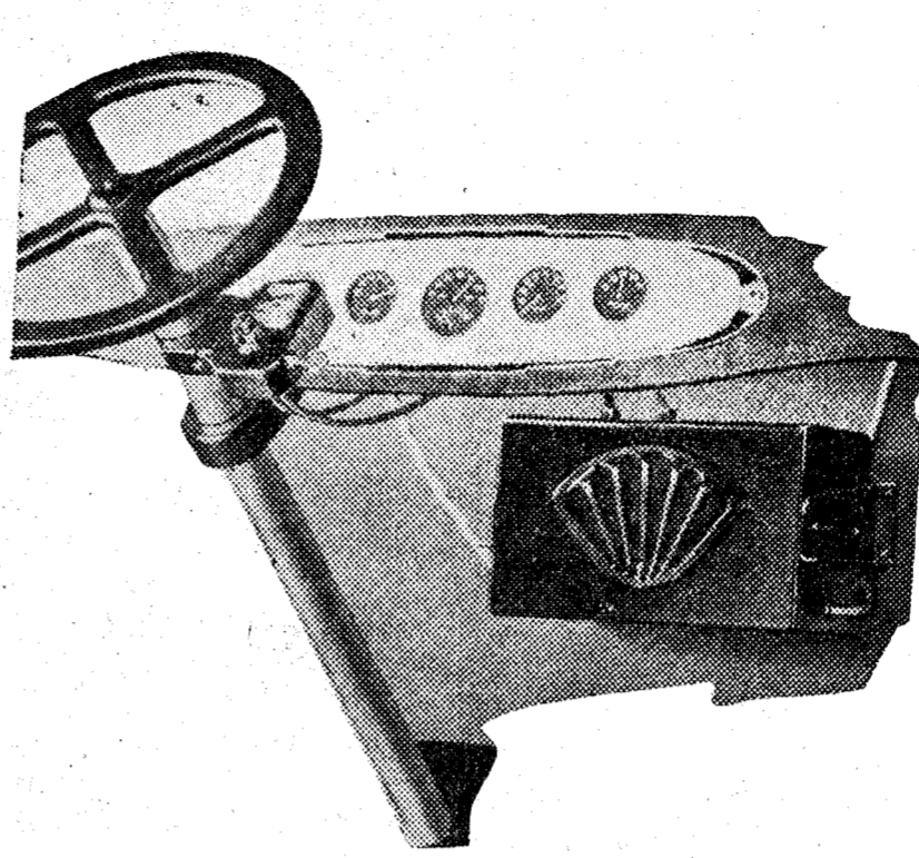
Equipo de Radio para automóvil Wells-Gardner, instalado por Teleaudió, Eduardo Dato, número 11, especializada en estos equipos
