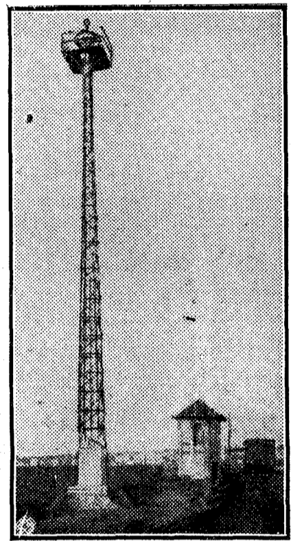
Castillete de iluminación instalado por la Casa Siemens en la Playa de Madrid
