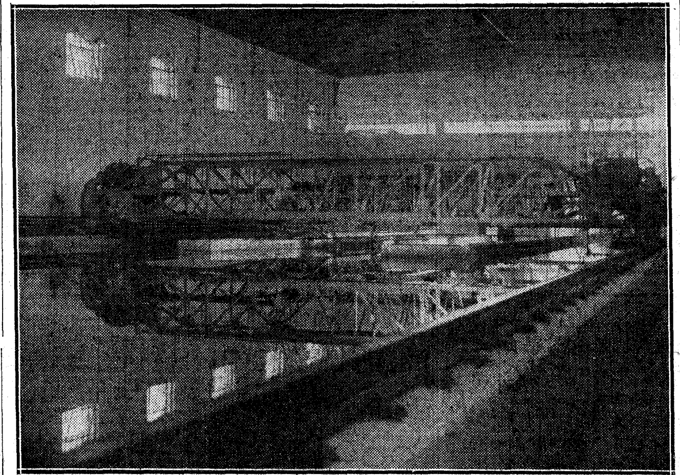
El carro de carga, que se mueve sobre raíles por encima del agua, al unísono de los modelos de barcos sujetos a prueba. En él se sitúan los observadores. Aparece reflejado en el agua, imperceptible ésta por un efecto de luz. La fotografía se ha obtenido cuando el carro estaba parado al comienzo del Canal. Pueden alcanzar velocidades de seis metros. (Fot. Sánchez del Pardo)
