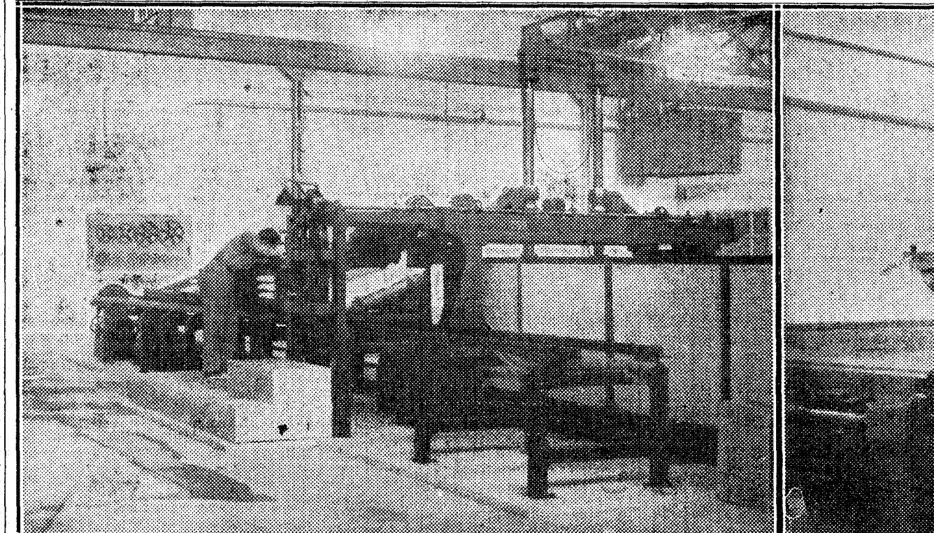
Puesto de mando de la máquina que talla las líneas de los modelos. Se dirige la máquina sin más que atender a un elipse, que franquea las líneas de un plano dibujado en mármol para evitar errores mínimos que puede producir la contracción del papel
