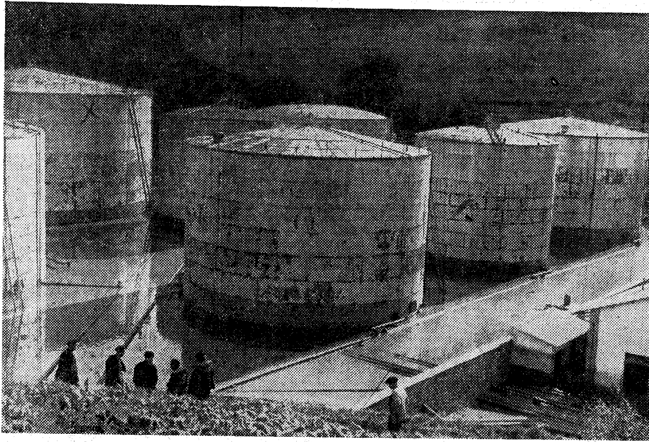
Los depósitos de la Campsa en Pasajes durante la inundación. Por efecto de ella, los tanques se inclinaron, se rompieron las tuberías y la gasolina se derramó. Durante varias horas existió el peligro inminente de un fuego gigantesco
