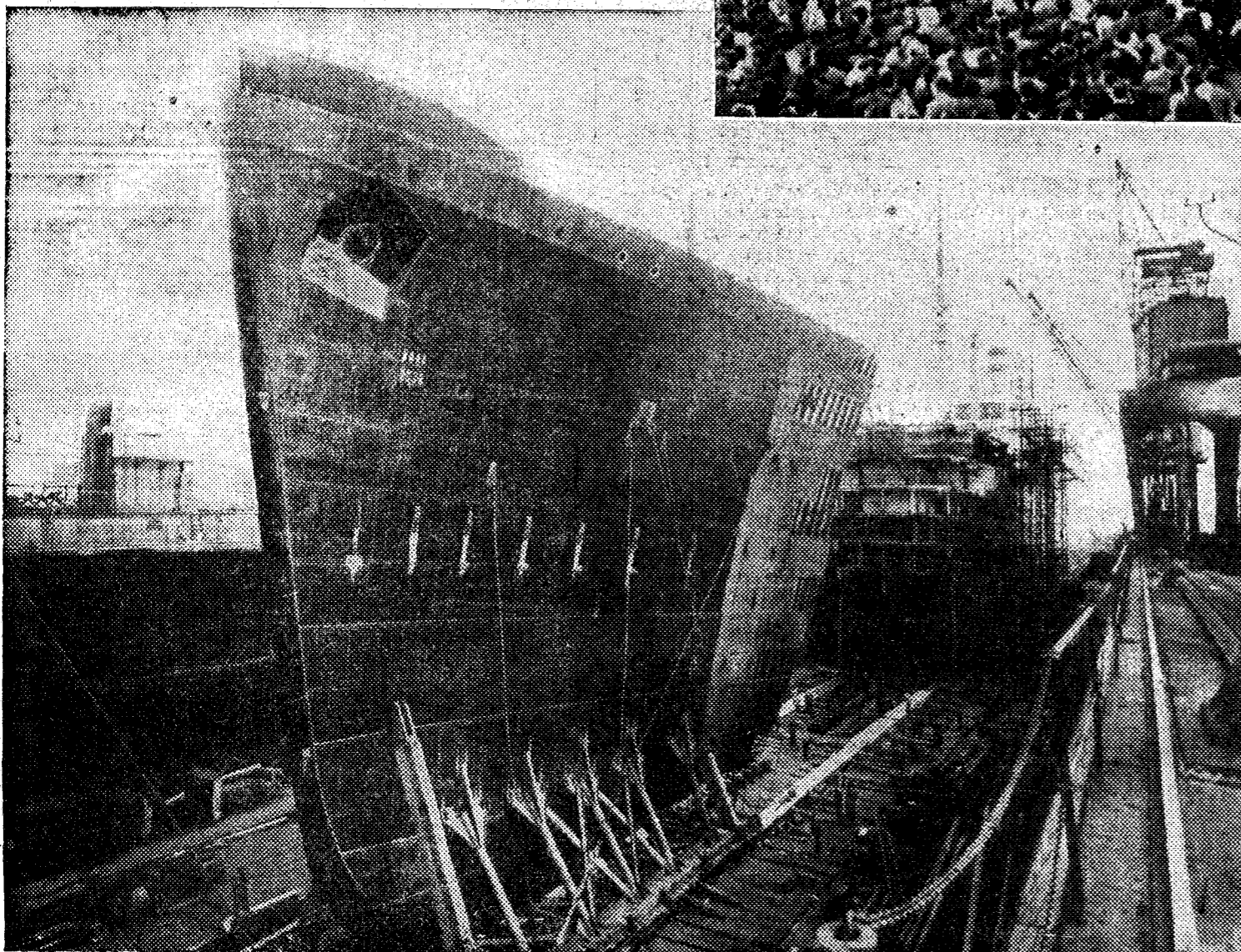
Abajo: Los trabajos de alargar el trasatlántico alemán "Hamburgo" en el puerto de Hamburgo. En la "foto" puede verse el corte efectuado en el gigantesco barco para alargarle 12 metros. El exterior del buque será modernizado
