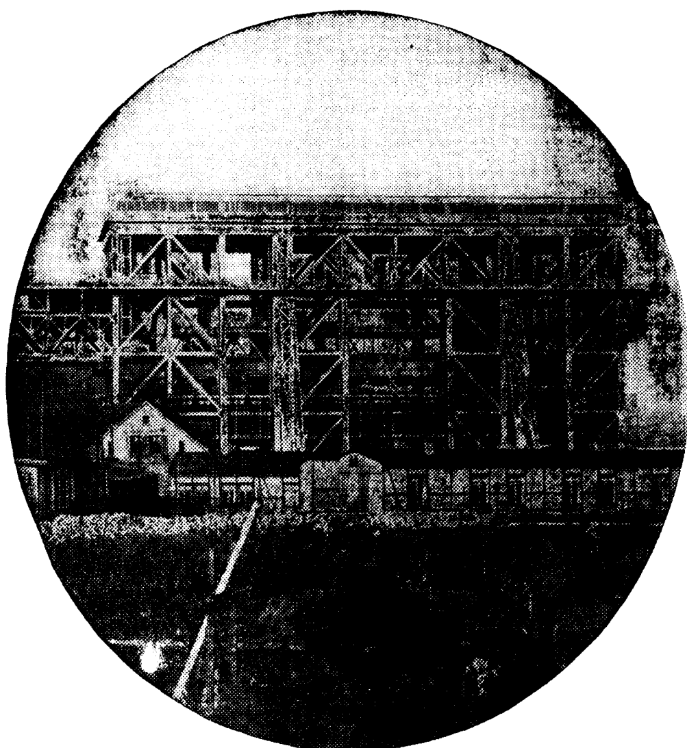
Una vista del gigantesco barco trasbordador que cruzará el Canal de Hohenzollern, y que podrá soportar 4.000 toneladas
