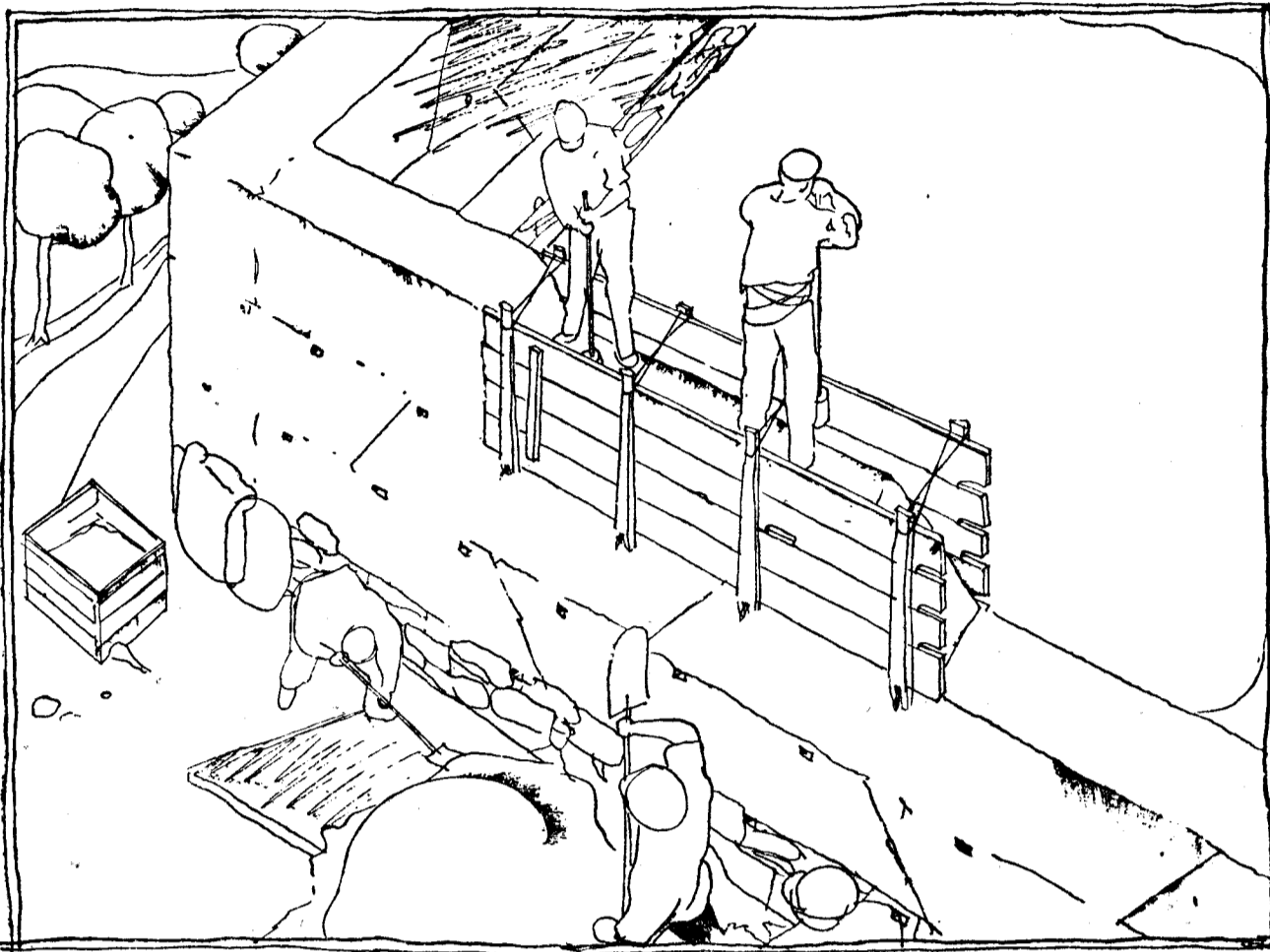
Esquema demostrativo de la técnica del tapial. Cinco hombres constituyen una cuadrilla de trabajo para cada tablero. Dos son apisonadores, otro amasador y dos peones (cavadores). Su rapidez es característica. Puede calcularse que ejecutan ocho metros cúbicos en la jornada de ocho horas
