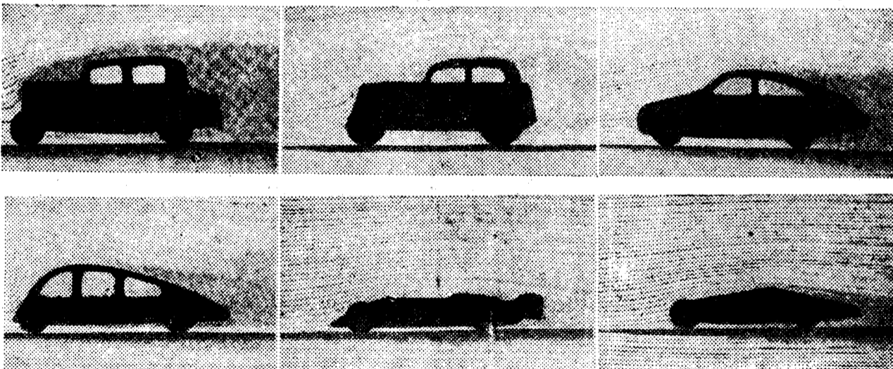
Ensayos por inyección de líquidos coloreados. Contrastan los torbellinos que corresponden a las formas ordinarias, con las penetraciones uniformes de las carrocerías aerodinámicas
