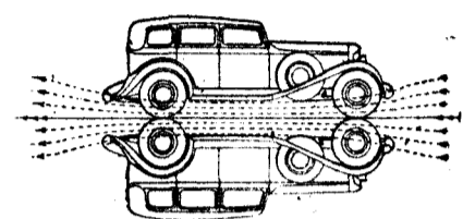
Medida de la resistencia del aire por el método de las imágenes
