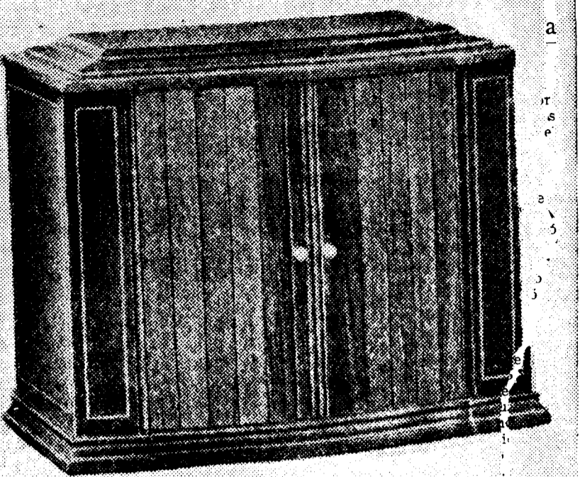
El célebre Emerson 6 para onda corta y larga de 200 a 2.000 metros. Bellísimo mueble con puertas correderas. Lleva 6 lámparas de los últimos modelos, tres 78, una 6B7, una 43, una 25Z5. Dos pasos de radio frecuencia, dos pasos de frecuencia intermedia. Control automático. Dial iluminado calibrado en kilociclos. Funciona perfectamente para todas las audiciones nacionales y extranjeras sin antena ni tierra. Distribuidor para España: Radio Saturno, de Barcelona, y en Madrid: Isaac Martín, Churruga, 1.
