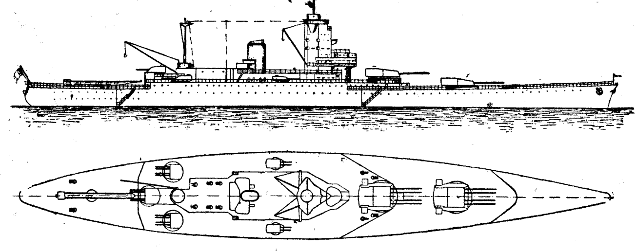
Plano del acorazado francés "Dunkerque", planeado para hacer frente a los acorazados de bolsillo alemanes tipo "Deutschland". El "Dunkerque" desplazaría 26.500 toneladas, andará 30 nudos y llevará ocho cañones de 330 mm. en dos torres cuádruples a proa.
