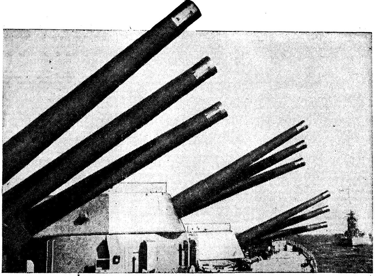
Los cañones de gran calibre del "Rodney". Nueva de 400 mm. en tres torres a proa del barco, que, con su gemelo el "Nelson", son los acorazados mayores del mundo. Llevan, además, 12 cañones de 152 mm. y cuatro anti-aéreos. El "Rodney" y el "Nelson" desplazan alrededor de 35.000 toneladas (Foto "Illustrated London News".)
