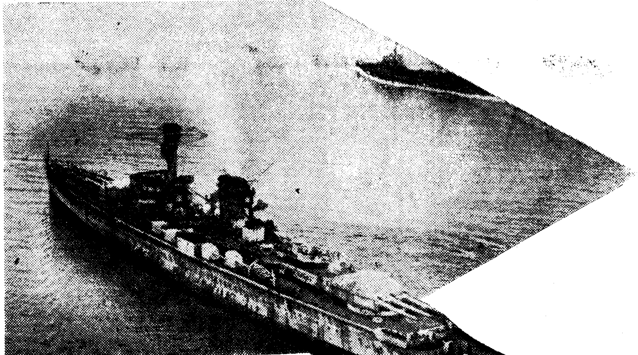
El "Deutschland", primero de una serie de cuatro buques iguales proyectados—uno ya en servicio y otro en construcción muy adelantada—por Alemania para poseer acorazados de acuerdo con las limitaciones impuestas por el Tratado de Versalles. El "Deutschland" desplaza, pues, 10.000 toneladas, anda 27 nudos y lleva seis cañones de 280 mm. y ocho de 150 mm.
