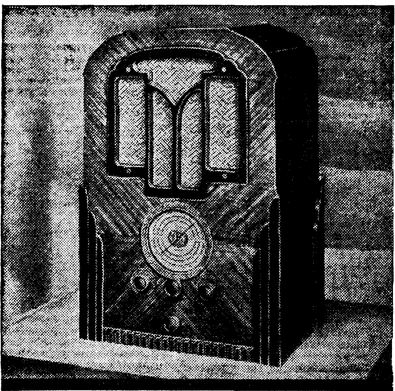
Superheterodino "B" ROA de 8 válvulas para ondas cortas (6.000 a 16.000 kcs.) y normales 500 a 1.500 kcs. Abarca las emisiones de broadcasting de 19, 25, 31 y 49 metros, las de aficionado, policía, avión, las normales de radiodifusión (200 a 550 metros) y largas (1.000 a 2.000 metros). El cuadrante de tipo de aviación, puede accionarse a dos velocidades, expresadas por las relaciones 9 a 1 y 55 a 1. Va equipado con control automático de volumen, control de color de tono, altavoz dinámico y funciona con corriente alterna 115 voltios, 50 períodos. Demostraciones: Eduardo Dato, 9.
