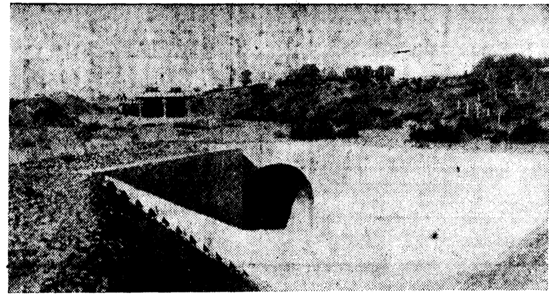
Sifón para el paso del arroyo Garcí-Pérez, de 3 m. de diámetro interior y 75 m. de longitud
