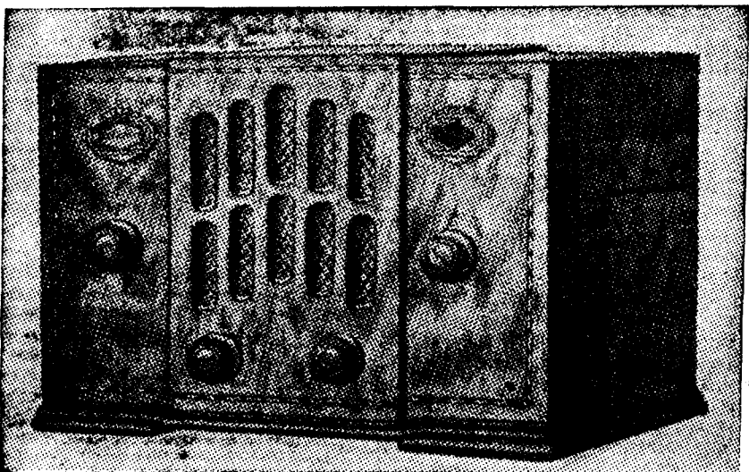
Aspecto del nuevo modelo CLEARVOX UL-6, de ondas de 200 a 2.000 metros y 6 válvulas ultramodernas, que acaba de lanzar a la venta la conocida y acreditada Casa Radio Popular, Desaguado, 14.
