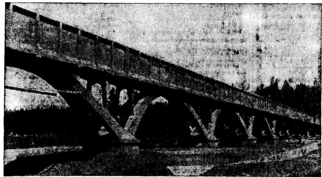
Acueducto sobre el arroyo Almonaza, con arcos de 18 metros de luz
