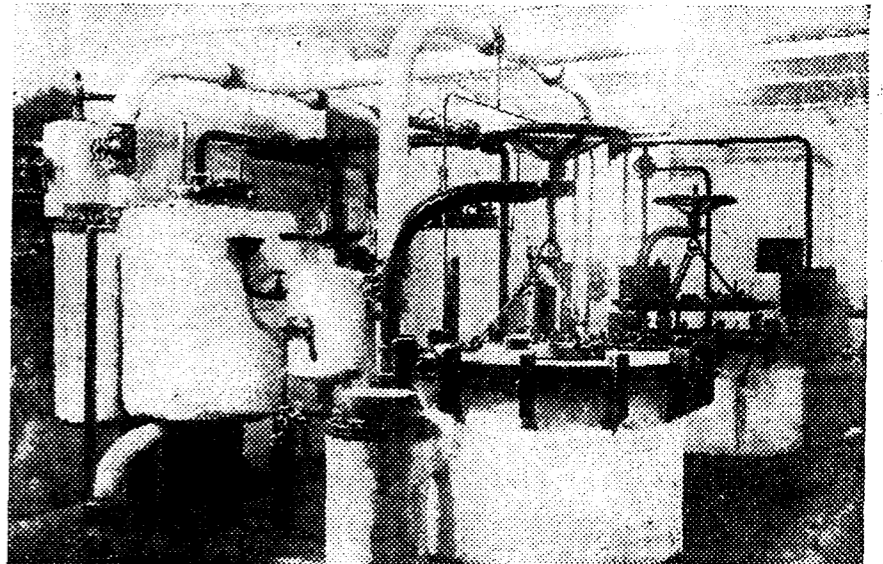
Instalación de impregnación de la fábrica de condensadores MANENS, Societá Scientífica Radio, S. A., Bolonia, Italia, representada en España por Empresas Radio-Eléctricas, S. A., Peligros, 2, Madrid.
