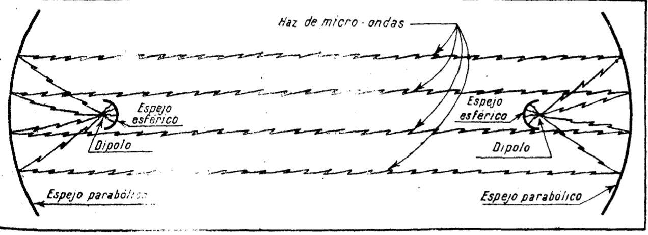
Fig. 1.— Sistema electro-óptico
