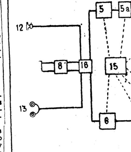
Fig. 3.— Esquema de una estación terminal.—1) Modulador. 2) Demodulador. 3) Control de la transmisión. 4) Id. de la recepción...
