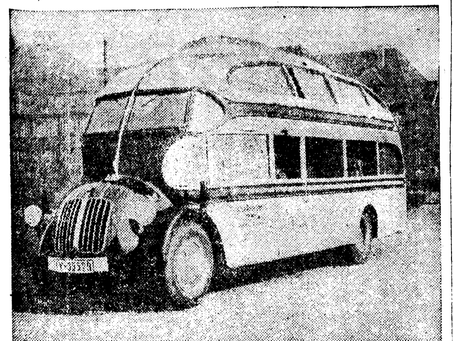
El autobús "Aero", que circula entre Essen y Berlín, con una velocidad media de 80 kilómetros por hora. Forma aerodinámica muy acusada y construido casi todo con aleaciones ligeras. Pesa la caja 380 kilos, correspondiendo 80 solamente a cada viajero
