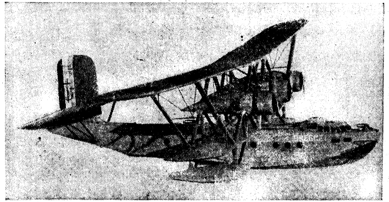
Hidroavión Breguet "Bizerta", construido por completo con aleaciones ligeras
