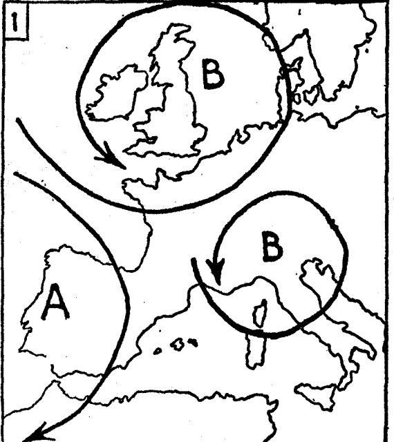
Distribución de las altas y de las bajas presiones barométricas alrededor de España, que es propensa a dar origen a vientos huracanados y temibles en la Península Ibérica. ¿Se presenta ahora?...
