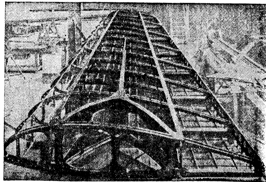
Armadura en duraluminio de avión metálico
