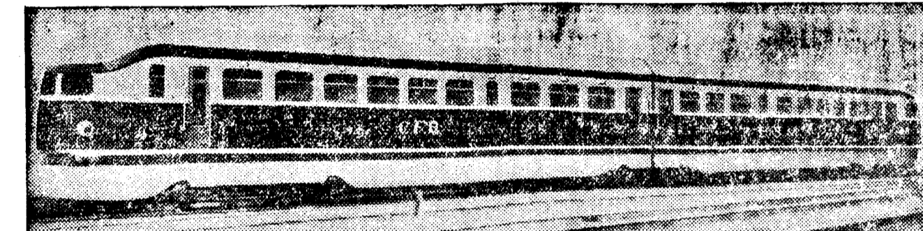
Autocarril Diesel-Maybac (ferrocarriles del Estado belga). Bastidor, motores y carrocería total en duraluminio
