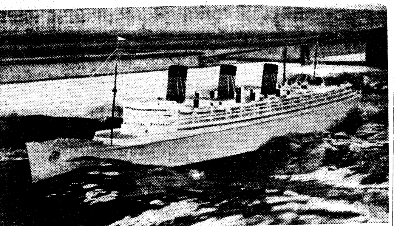
EL BARCO QUE NO SE ATREVIO A ASEGURAR EL LLOYD Maqueta, de seis metros, del gran trasatlántico en construcción de la Cunard "Queen Mary", de 70.000 toneladas, haciendo ensayos "en plena tormenta" en el tanque de pruebas. La primera dificultad que surgió, fuera la construcción, fué que, dado el coste del buque, los aseguradores del Lloyd no se atrevían a asumir todos los riesgos
