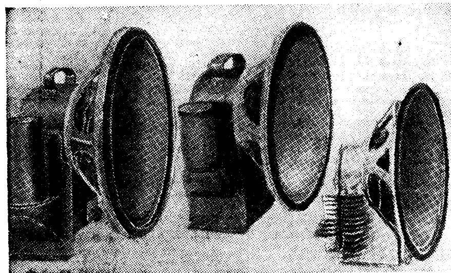
Los tres modelos de altavoces Jensen, Auditorium, Orthodinámico y Concert, que representa la Casa Dielectro, Paseo de Recoletos, 16
