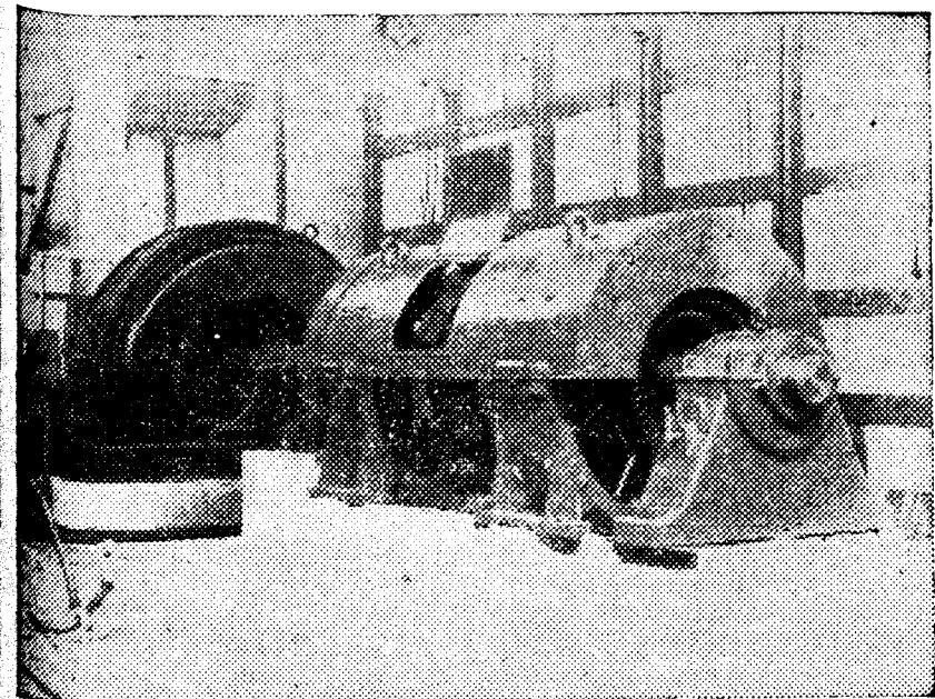
El motor de propulsión del "Artabro"; 500 caballos a 300 revoluciones
