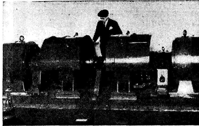
Los generadores y excitatrices del "Artabro", listos para las pruebas
