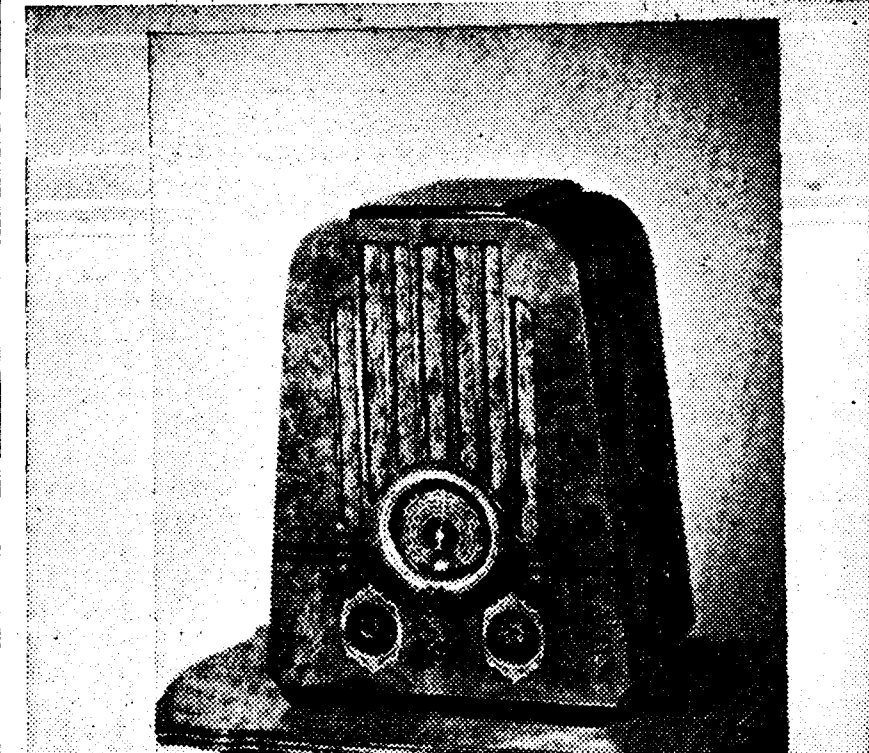
Ultramar modelo 1056. Radio receptor de 5 gamas para onda extra corta, corta, larga y extra larga. Alcance, desde 12 a 2.100 metros. Exclusiva: Sanz, Montera, número 29. Madrid
