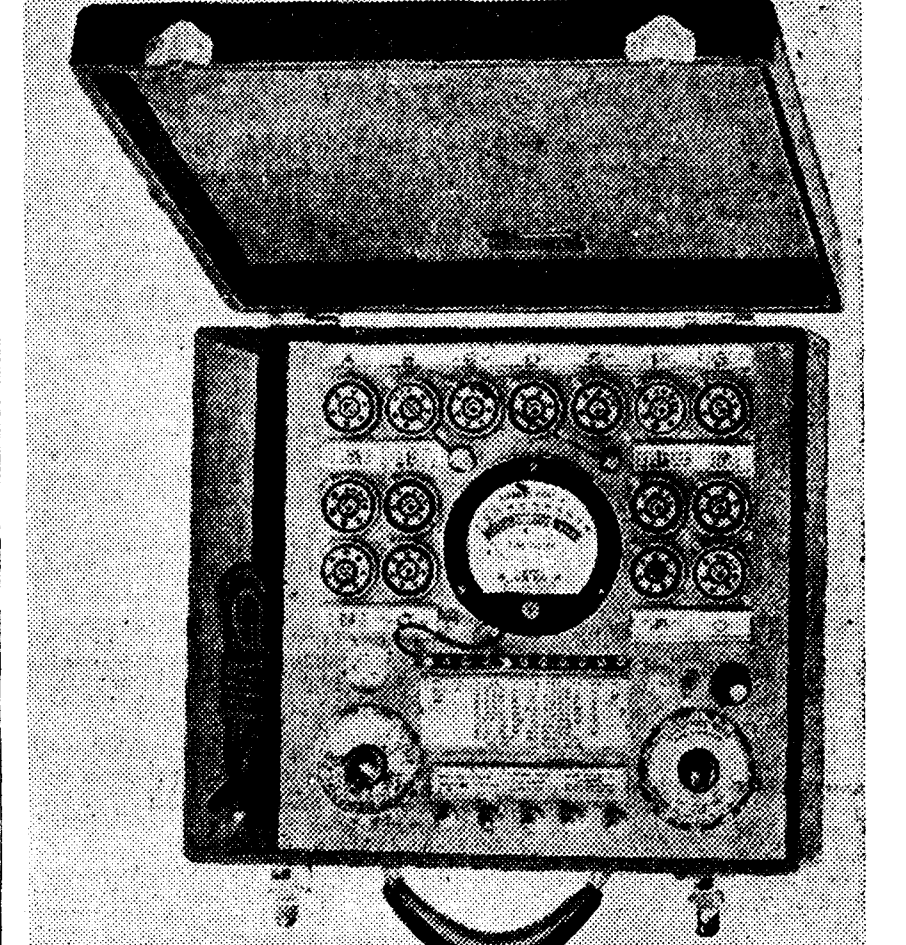
Corprobador de válvulas Diamond Point J 34 F, de la renombrada Casa Hickok, que fabrica como mayor especialidad toda clase de aparatos de comprobación de máxima precisión para fábricas y talleres de reparación de receptores de radio. Distribuidor exclusivo para España y sus colonias: Jaime Schwab, Los Madrazo, 6 y 8. Madrid
