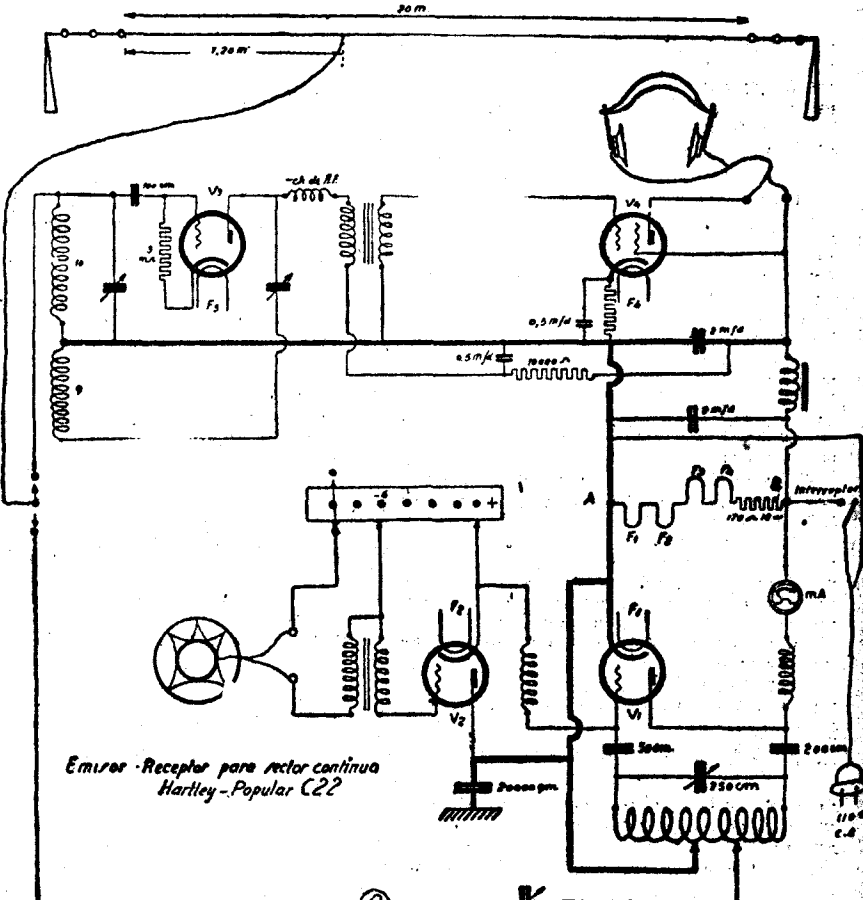
Reproducimos de la nueva revista "F. A. R." el esquema de una emisora-receptora para aficionados
