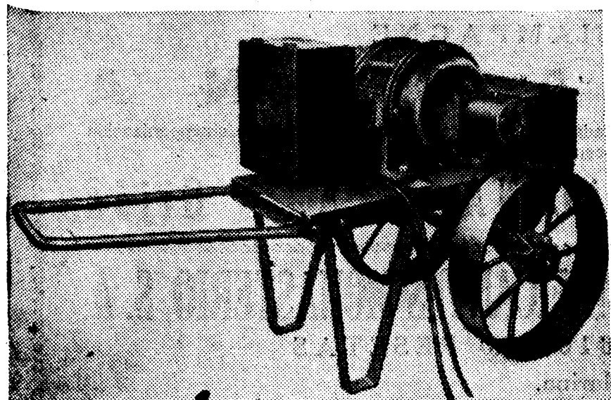
Equipo transportable formado por motor eléctrico, con transmisión para usos múltiples en las haciendas
