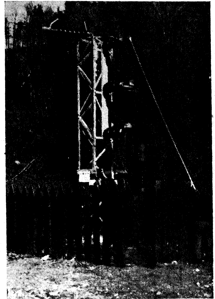
Subestación rural de transformación y distribución, 50 KVA., 66.000/2.300 volts., monofásica
