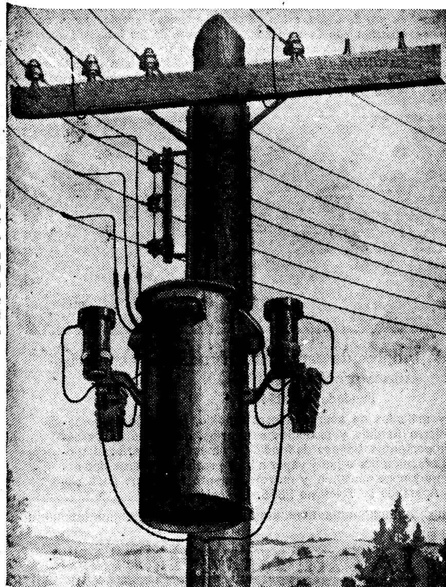
Subestación rural de transformación y utilización, 10 KVA., 2.300/220-110 volts., equipo completo montado sobre poste
