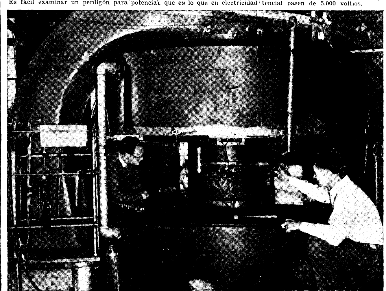
Los asistentes del doctor Lawrence colocando la caja que sirve de ametralladora para lanzar varios billones de deuterones por segundo, con una energía de algunos millones de electronvolts. La caja se encuentra entre las armaduras de un electroimán, de cuyas dimensiones gigantescas da idea la fotografía
