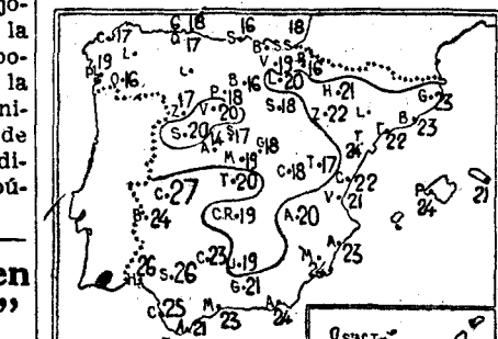
Temperaturas máximas del día 19
