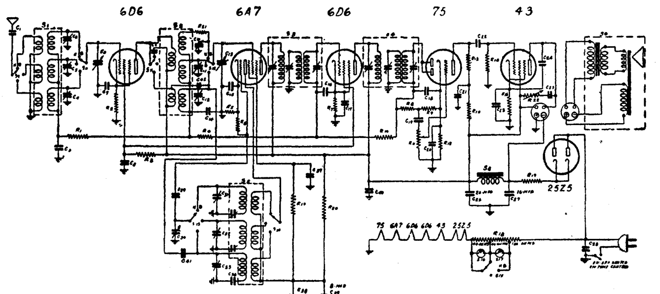
Diagrama esquemático del nuevo "Pilot", modelo 125, de la Casa Schwab
