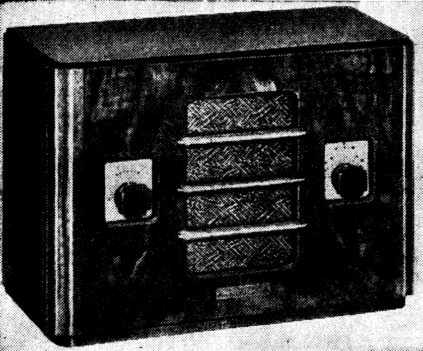
Modelo Westinghouse WR21B, superheterodino de 5 válvulas, universal, para ondas larga y normal, válvulas RCA. Dirijase a Vivomir, Alcalá, 67.
