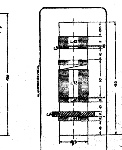
Otro detalle explicativo referente al esquema Tungsram para superheterodino de 6 válvulas, corriente alterna, todas ondas, publicado en nuestra página del 19 del pasado mes de noviembre
