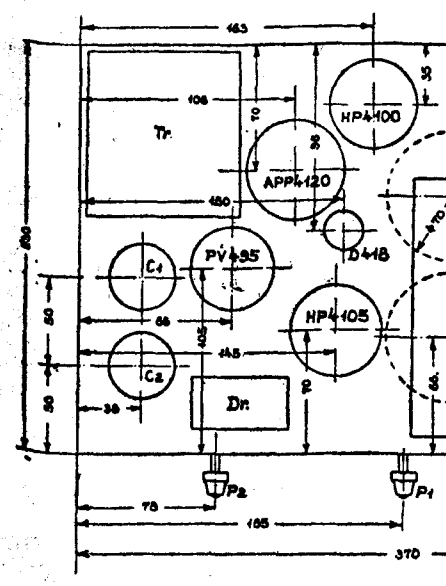
Publicamos la explicación del esquema Tungsram para superheterodino de 6 válvulas para corriente alterna, todas ondas, publicado en nuestra página del 19 del pasado mes. En la próxima publicaremos la lista de materiales.
