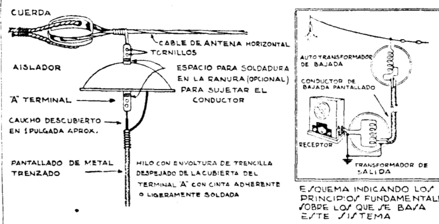
Dispositivo Statoformes, eliminador de parásitos, que distribuye Empresas Radio-Eléctricas, Peligros, 2
