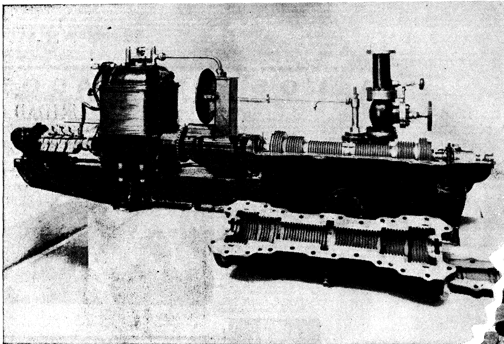
En este año cumple la turbina de vapor el medio siglo de vida. He ahí una de las primeras turbinas que Parsons construyó en 1886 (Foto Vidal)
