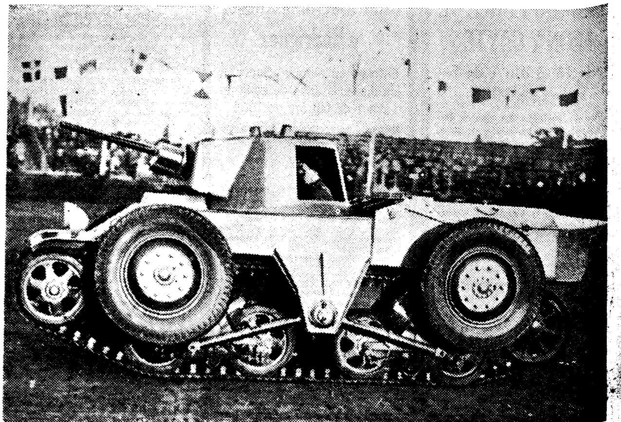
Un nuevo tanque sueco. En dieciocho segundos cambia el sistema de marcha. Sobre las ruedas alcanza una velocidad de 75 kilómetros, y de 40 como «auto-oruga» (Foto Vidal)
