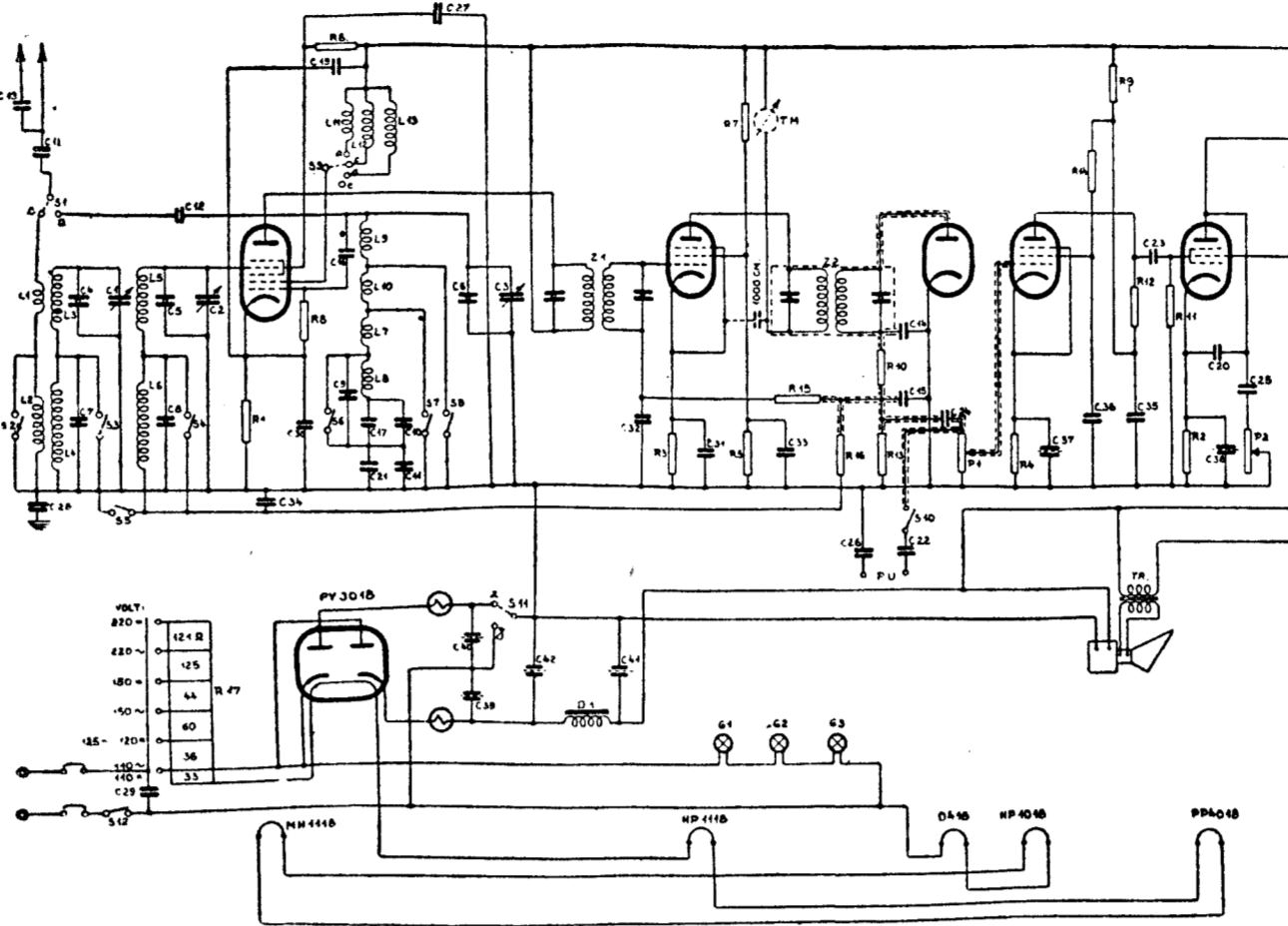
Esquema Tungram del superhet universal, toda onda, con regulación antifadig
