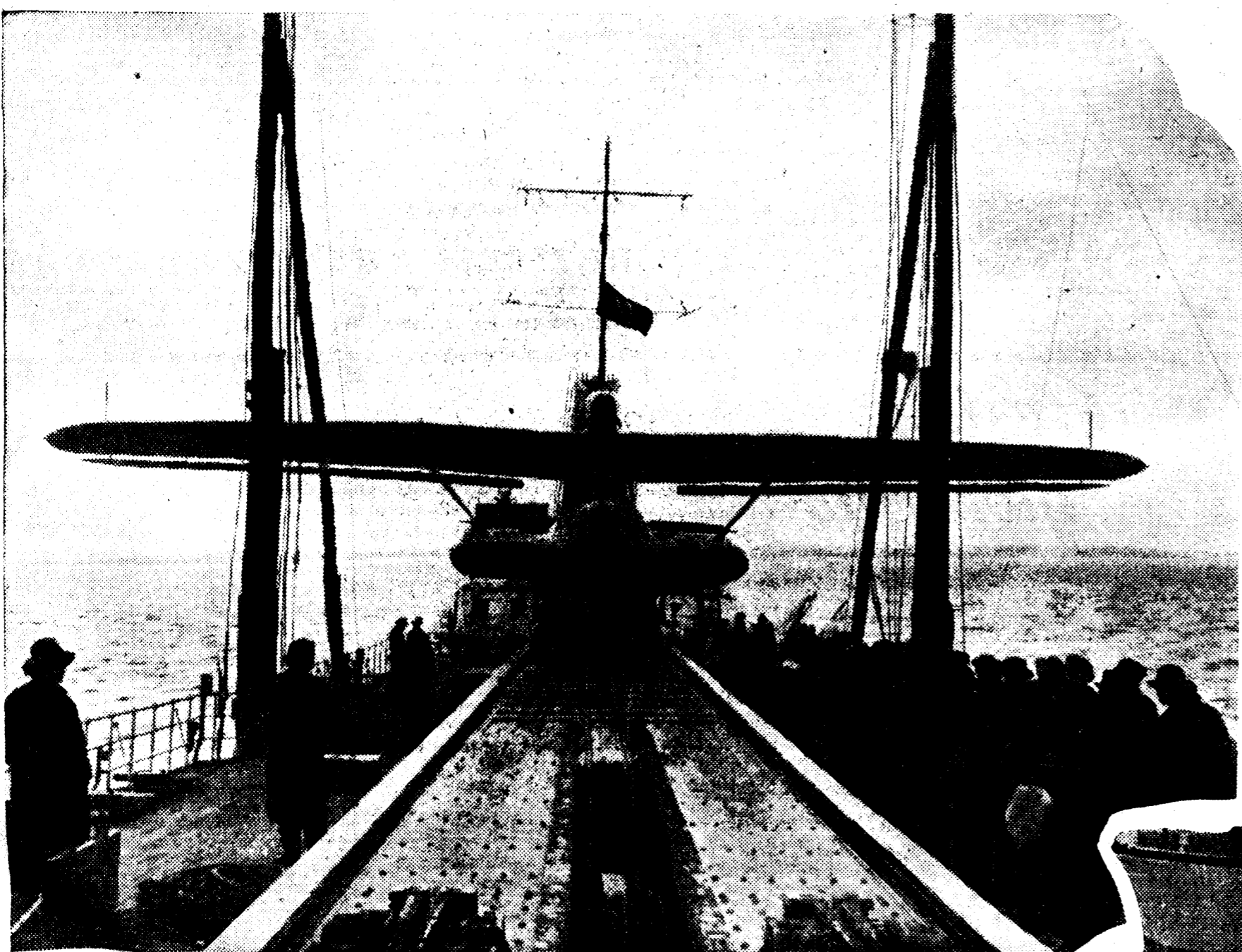
En Kiel (Alemania) se han hecho ensayos, coronados por el más halagador triunfo, de un nuevo sistema de catapulta para lanzar aviones desde la cubierta de los barcos; podemos ver aquí un momento de la impresionante maniobra. A la derecha, el tercer «aeródromo flotante» de Alemania, el «Ostmark», de Bremen, en el momento de iniciar su primer viaje experimental
