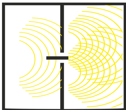
Ilustración 4.- Experimento de T. Young. Fuente: elaboración propia
