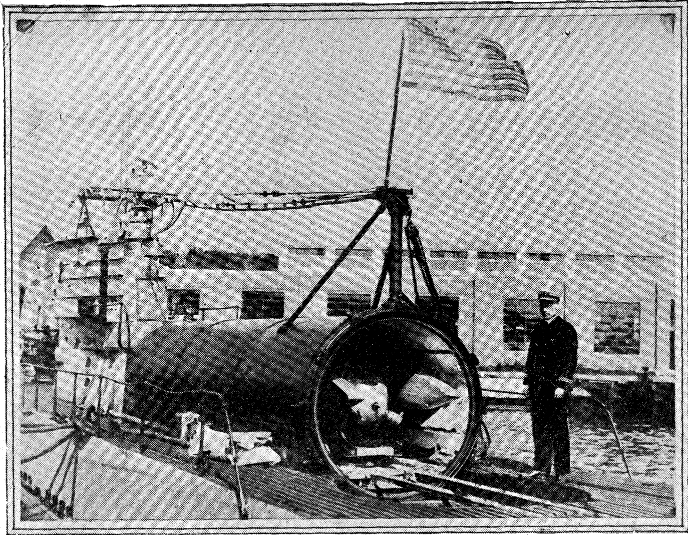
En los Estados Unidos se han realizado recientemente pruebas de un avión pequeño, que va colocado dentro de un cilindro impermeable sobre la cubierta de un submarino. Cuando éste se halla a flote el avión puede estar dispuesto para volar en el espacio de nueve minutos. (Fot. Vidal.)
