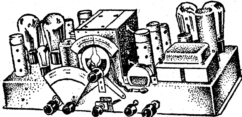
Formidable aparato "Kennedy" de doce válvulas, recién lanzado al mercado español por don José Briones, de Radio Popular
