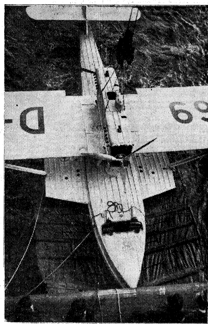
Un nuevo y original sistema de llevar aviones. El barco "Westfalen", de 5.000 toneladas, de la "North German Lloyd"
