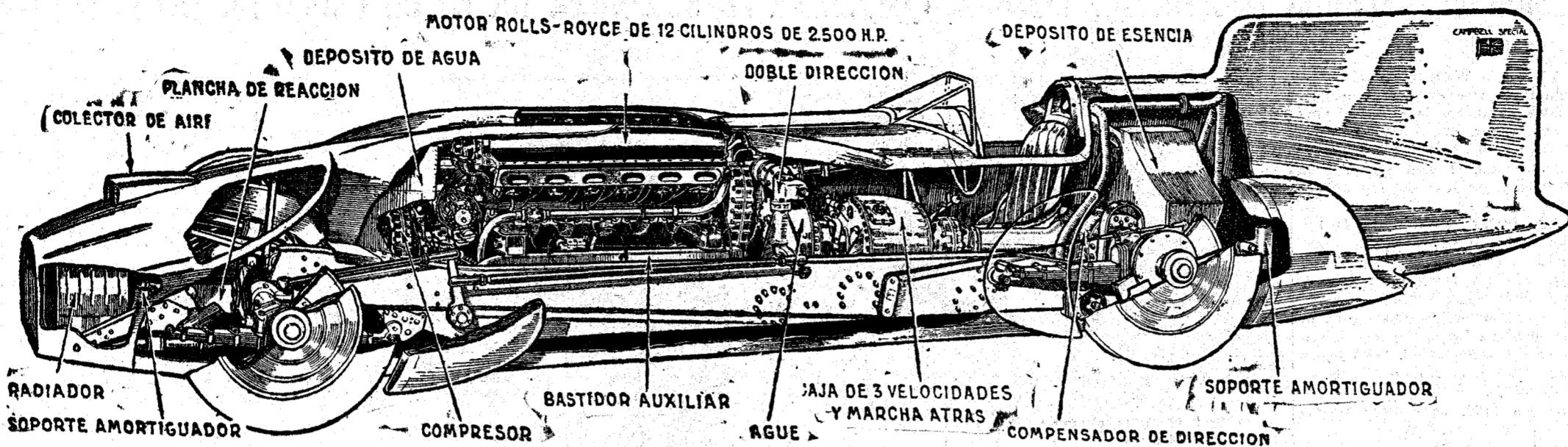
Un corte, dibujado en el estudio técnico de "The Motor", del "Pájaro Azul", con el que Sir Malcolm Campbell intentará alcanzar la fantástica velocidad de 450 kms. por hora.
