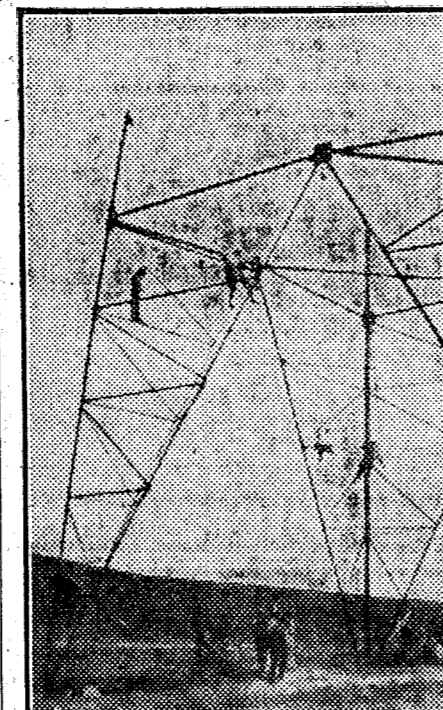
Uno de los mástiles autoestables en construcción para la emisora nacional portuguesa.
