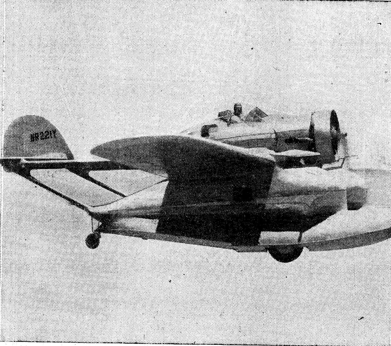
Aparato anfíbio construido para que el aviador norteamericano Charles Rocheville realizara un viaje de exploración por el río Mackenzie, con el fin de obtener películas documentales. Durante las pruebas en la bahía de Huntington, el avión capotó, y el piloto, al ser arrojado de la carlinga, cayó al agua y resultó con pequeñas heridas.
