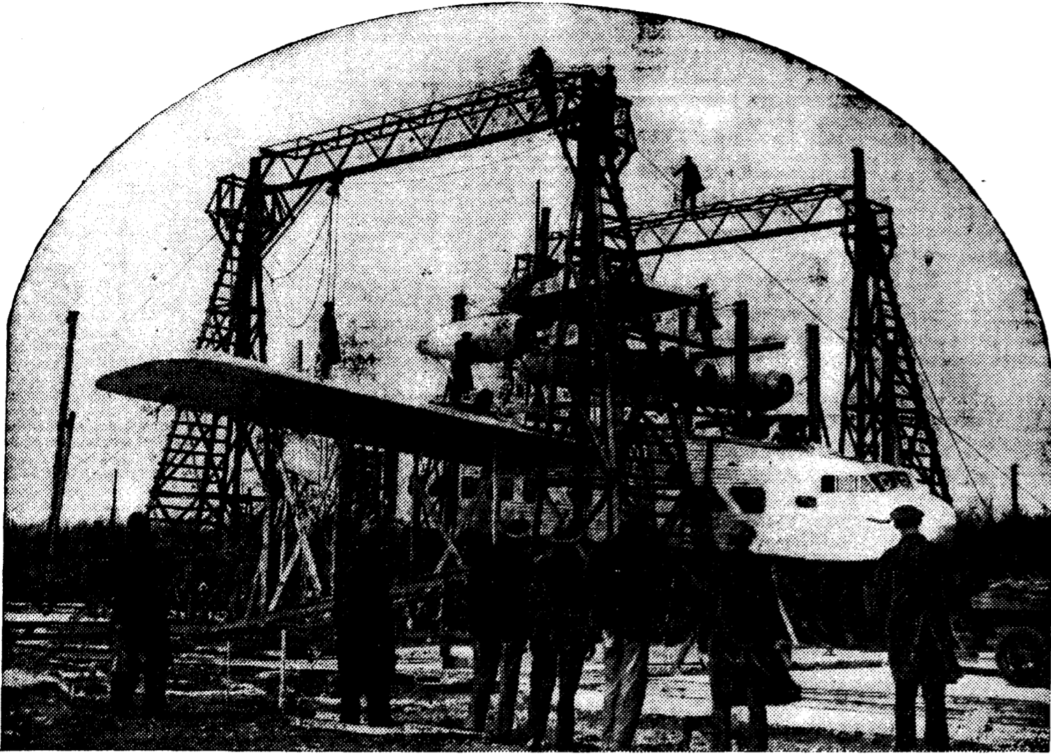
El "Scylla", este es su nombre, ha sido construido en Rochester y trasportado en piezas, por carretera, única manera que se ha podido emplear para trasladar este gigante. Tiene cabida para 39 pasajeros
