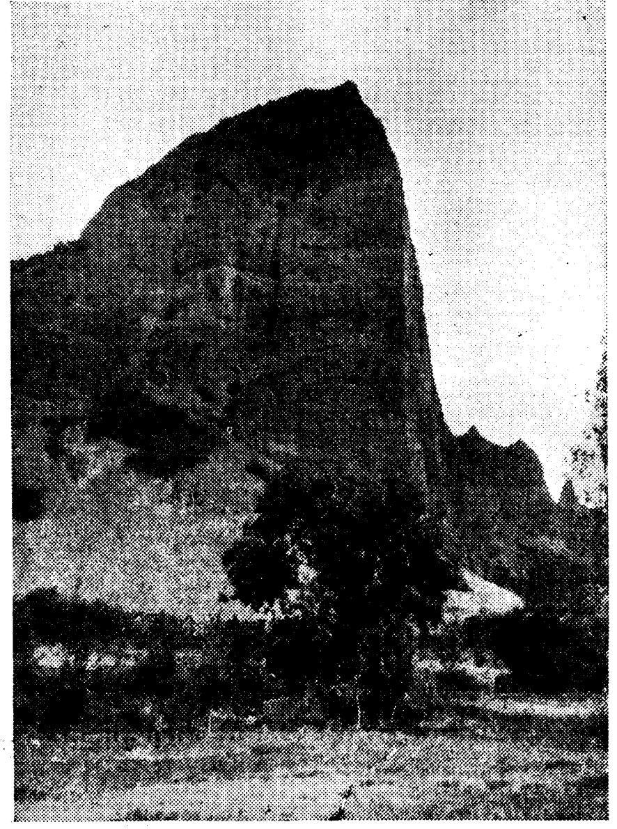
Las Médulas (León): vista de un tajo, en el que se observan las galerías romanas y la potencia del aluvión aurífero que beneficiaban. (Cliché propiedad del Consejo de Minería.)
