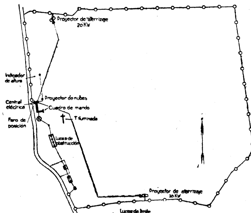
Plano general del aeropuerto nacional de Madrid, indicando la situación de todos los aparatos que constituyen el equipo completo de iluminación y señales
