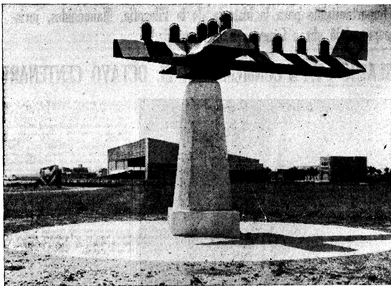
T indicadora de la dirección del viento, con catorce luces verdes de 100 voltios
