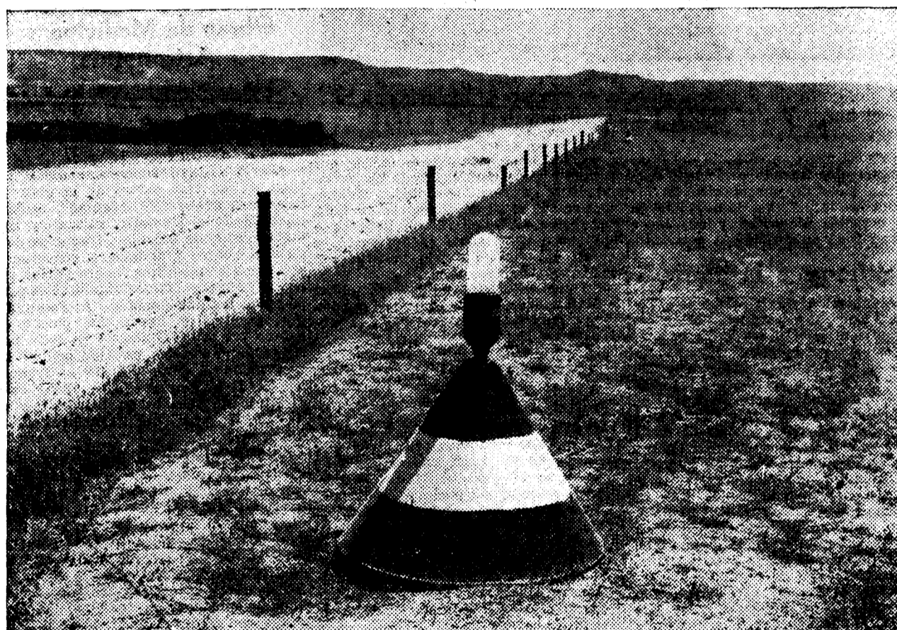
Luz de límite de 1.000 lumens (145 W.), montada sobre su cono
