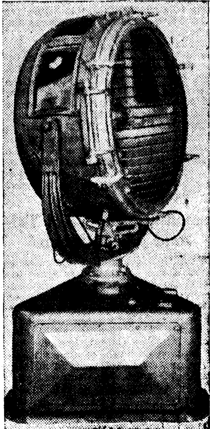
Faro de posición de veinticuatro pulgadas, dos millones de bujías, lámpara de 1.000 Wts. 30 voltios
