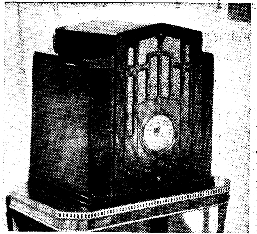
RECEPTOR WESTINGHOUSE WR-45, gran superheterodino, de ocho lámparas, para TODAS ONDAS, extra-corta, normal y larga. Altavoz electrodinámico de 8". Tonalidad absolutamente perfecta, gran potencia y sensibilidad finísima. Amplificación clase B. Control de tono. Control automático de volumen. Cuadrante tipo "Aeroplano". Capta todas las estaciones del mundo. Su mueble precioso es de una resonancia perfecta. Conexión para fonógrafo. Distribuidor: P. E. M. Vivomir, S. A. Alcalá, 67.—Madrid.
